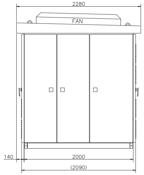
右側面図
