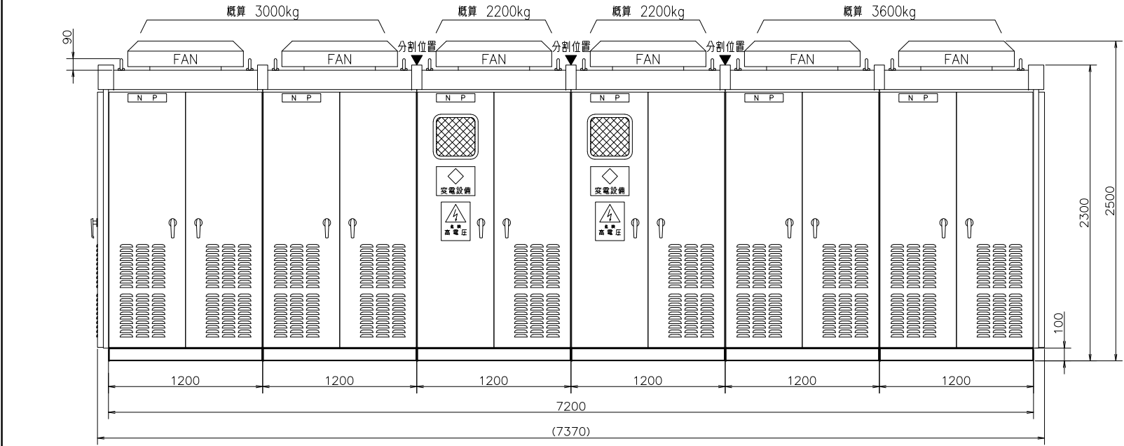
正面図
