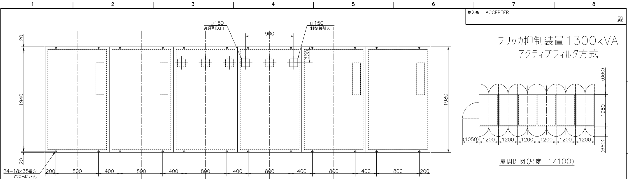
基礎図
