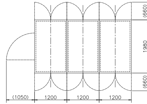
扉開閉図 (尺度 1/60)
