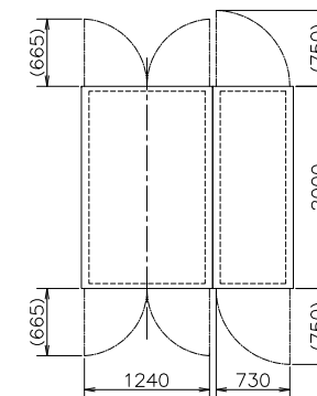
扉開閉図(尺度 1/60)
