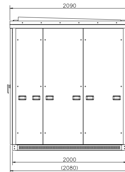
右側面図
