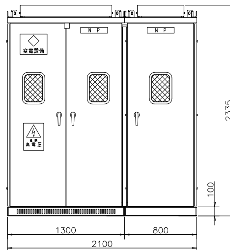
正面図
