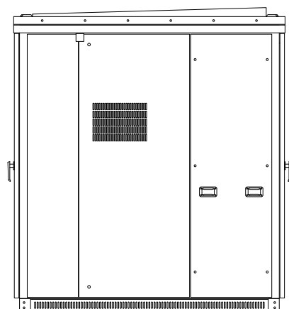
左側面図
