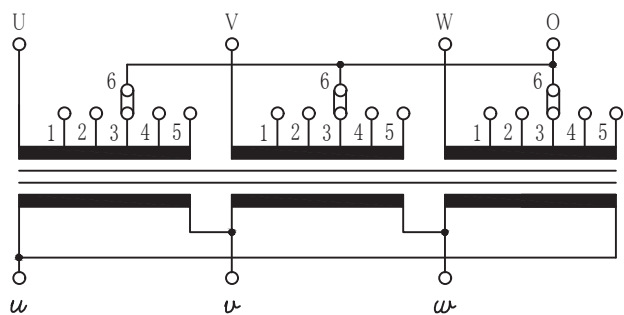
結線図
