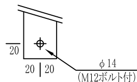
一次側端子 (t4×40)
