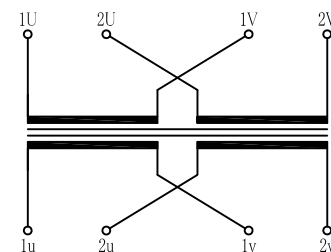
結線図
