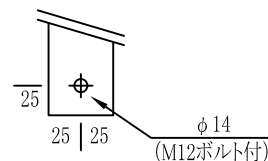
二次側端子 (t6×50)
