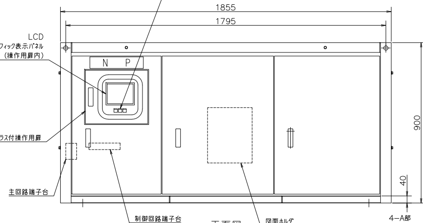
正面図
