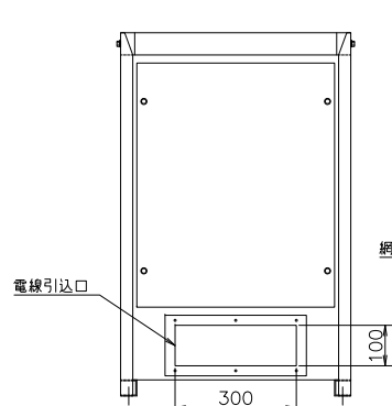
左側面図
