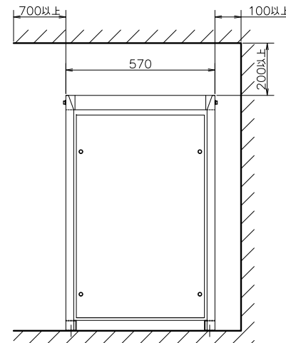
右側面図
