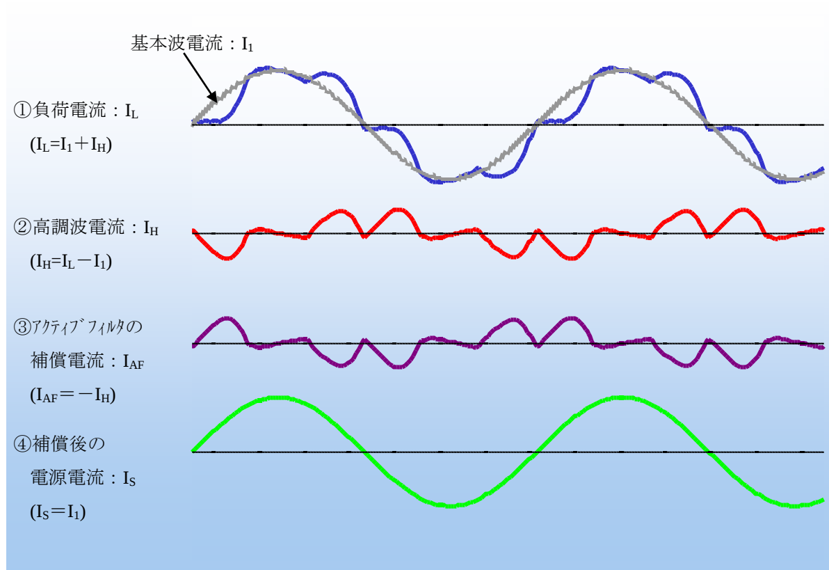
図 11 高調波補償動作原理
