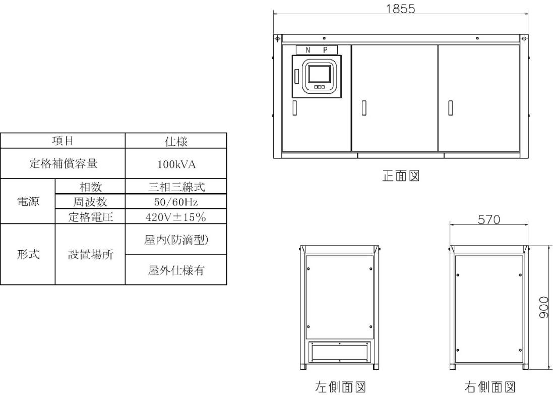
図 12 アクティブフィルタの仕様および外形寸法
