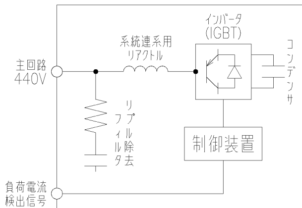
図 10 アクティブフィルタの構成
