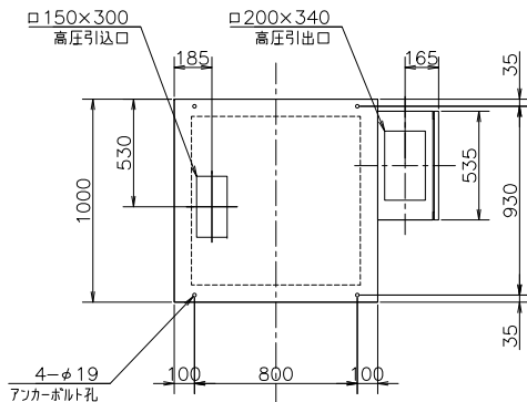
基礎図
