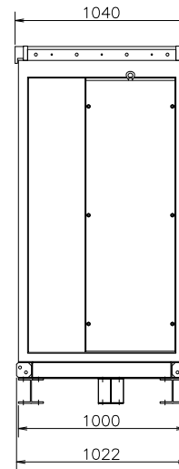
右側面図
