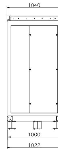
右側面図
