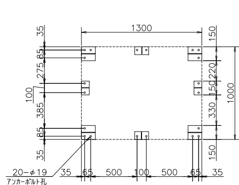
H鋼基礎図
