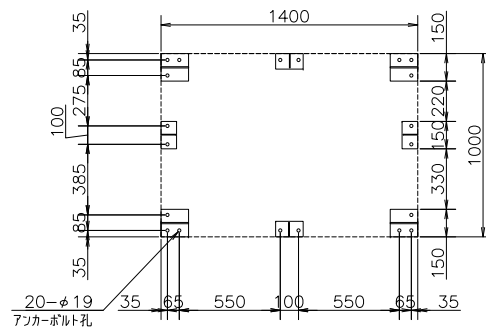
H鋼基礎図
