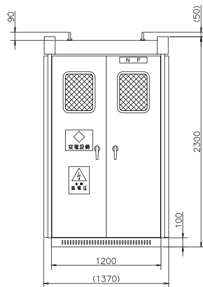
正面図
