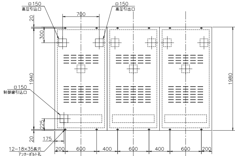
基礎図
