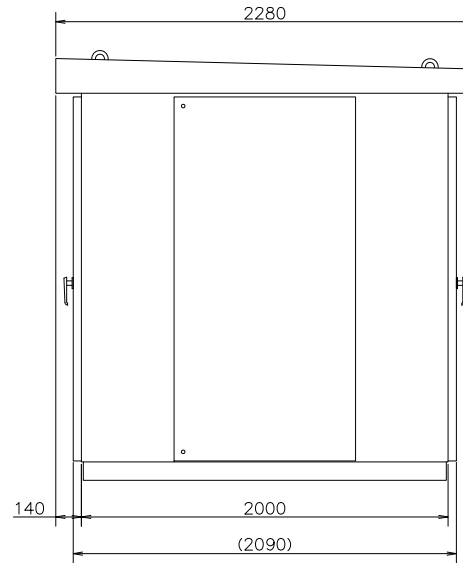
右側面図
