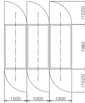
扉開閉図 (尺度 1/60)
