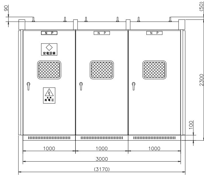
正面図
