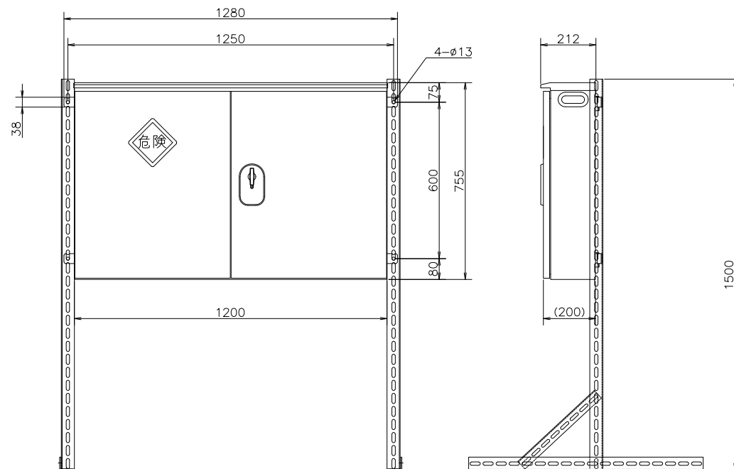
正面図
