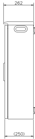
右側面図
