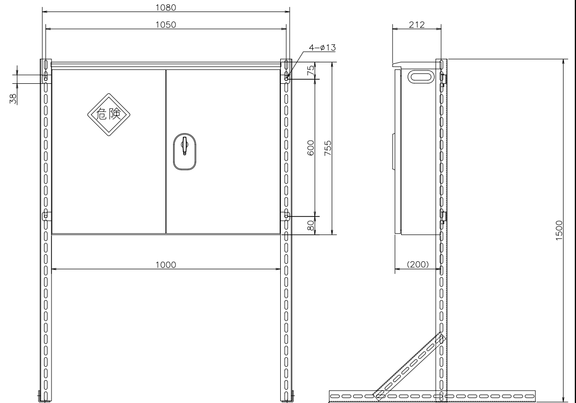
右側面図
