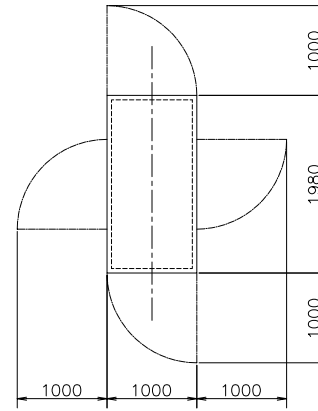
扉開閉図(尺度 1/60)
