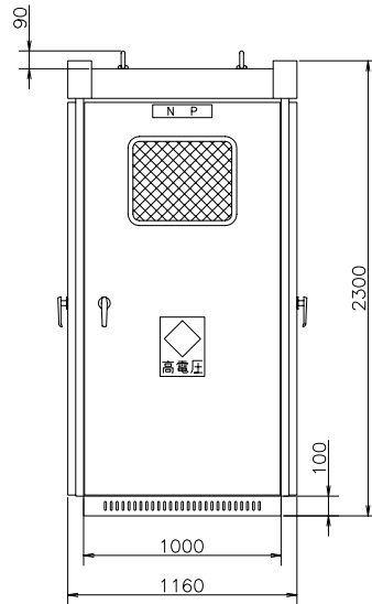
正面図
