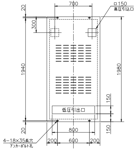
基礎図
