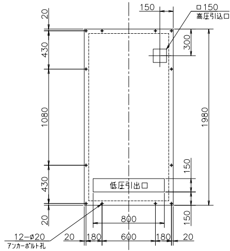
基礎図
