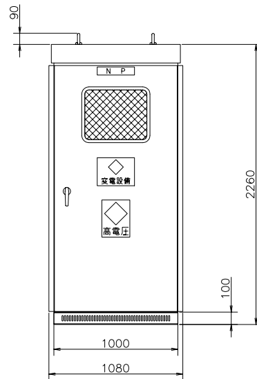
正面図
