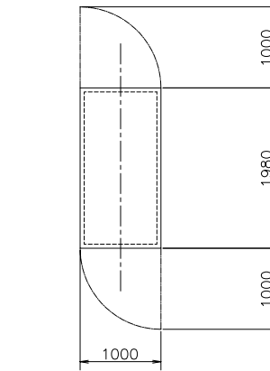
扉開閉図(尺度 1/60)
