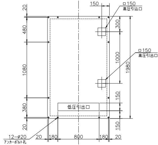
基礎図
