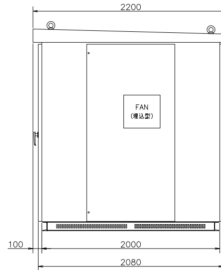
右側面図
