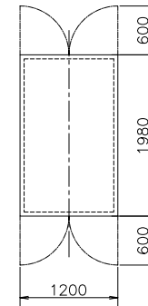
扉開閉図(尺度 1/60)
