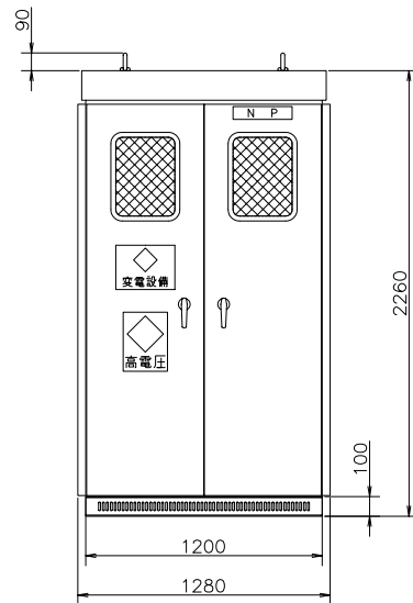
正面図
