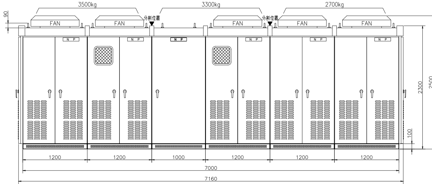
正面図
