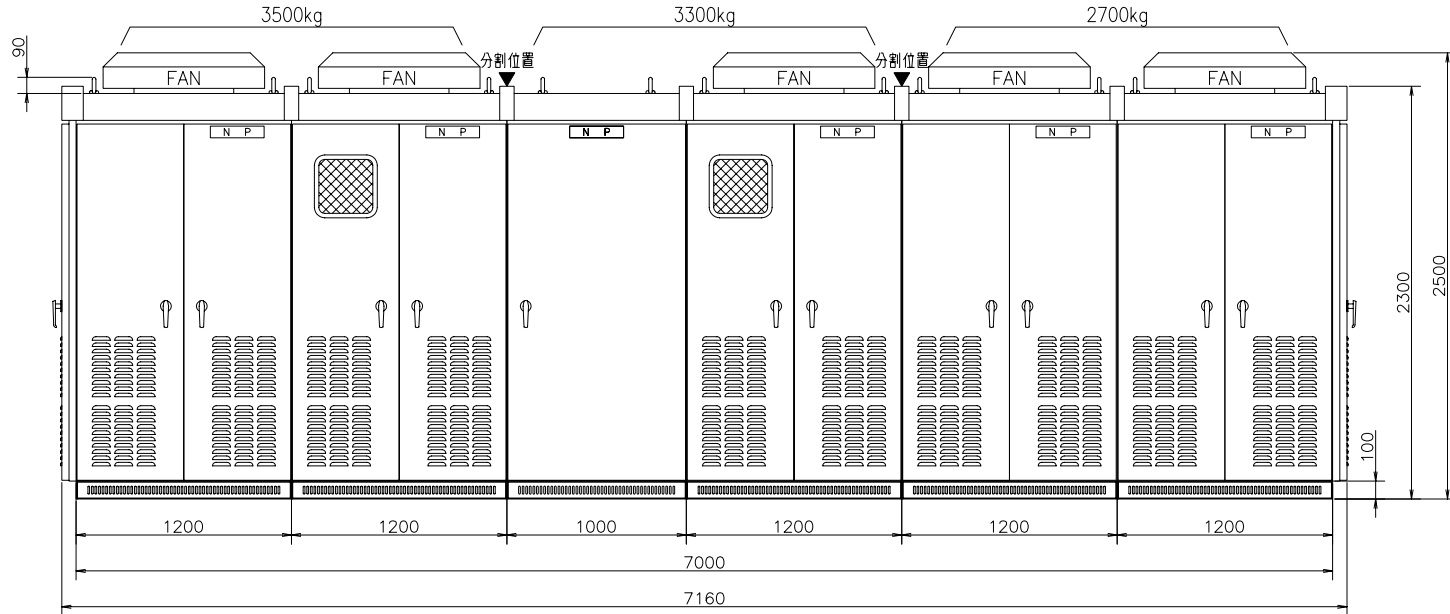
正面図
