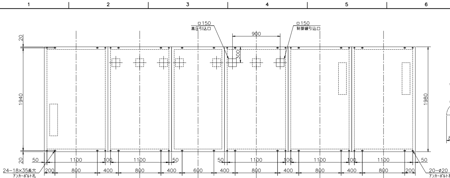
基礎図
