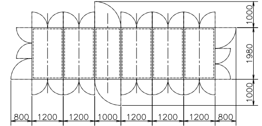
扉閉開図(尺度 1/100)
