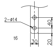
端子詳細図 (引込引出部分) (尺度 1/6)
