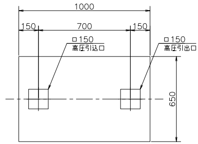
底面図
