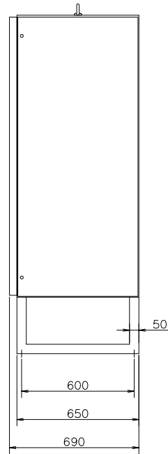
側面図
