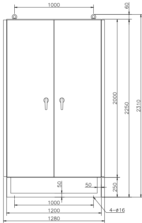
正面図
