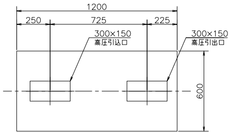
底面図
