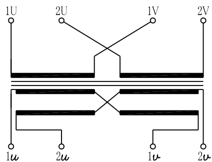
結線図
