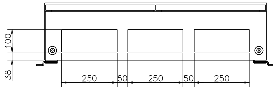
底面図
