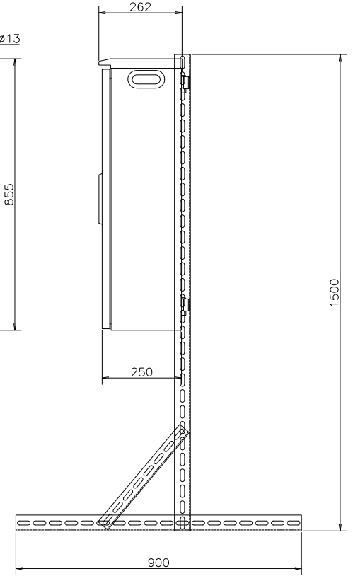
右側面図
