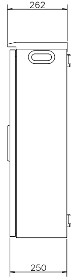
右側面図
