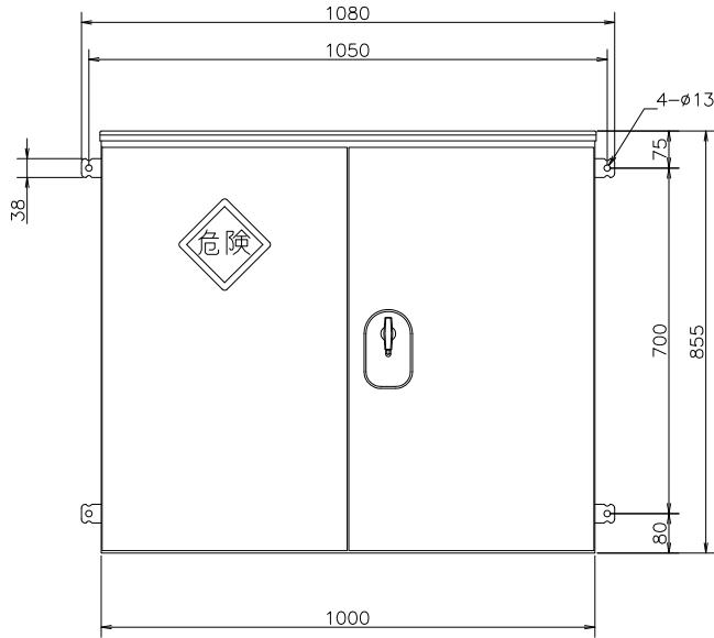
正面図
